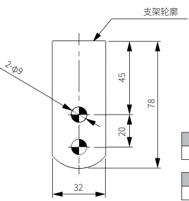
L型支架
