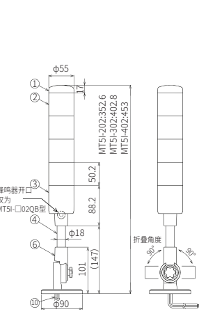
折弯底座
