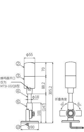
L型支架
