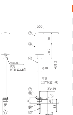
MT5I-102L□J
