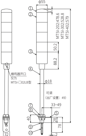
MT5I-□02L□J
