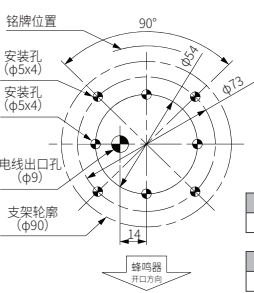
折弯底座
