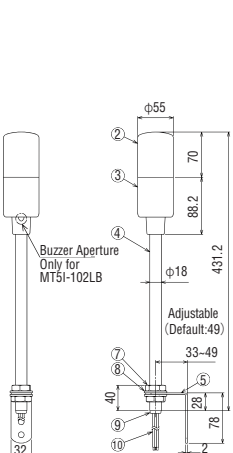
MT5I-102L□J
